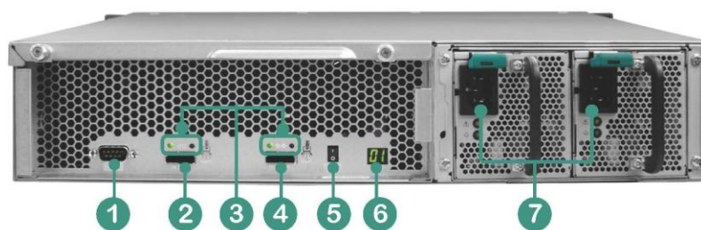
REXP-1200U-RP
