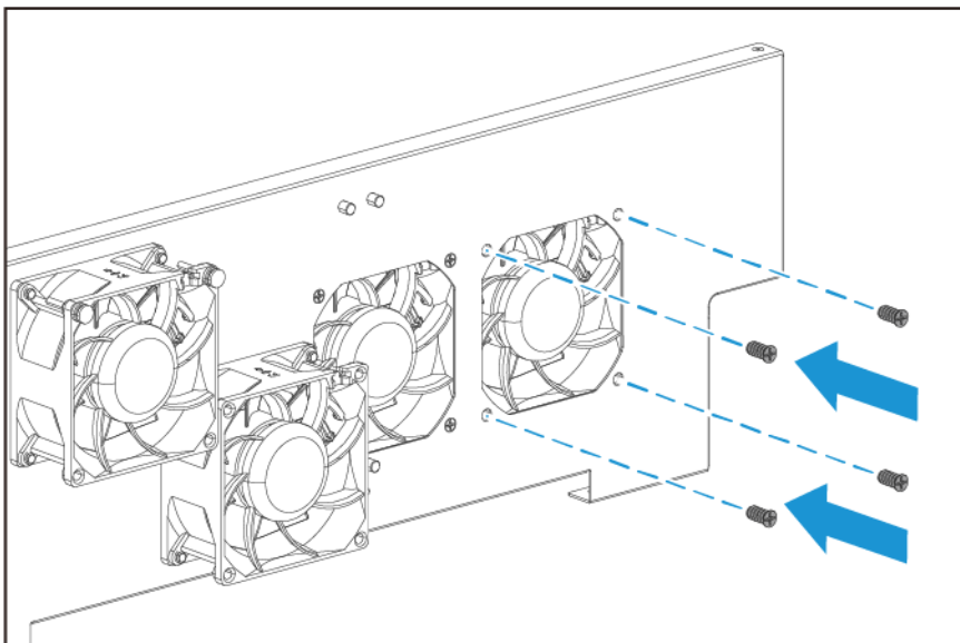
시스템 팬
