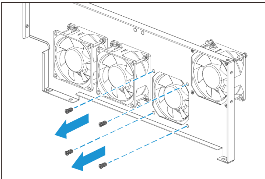
CPU 팬
