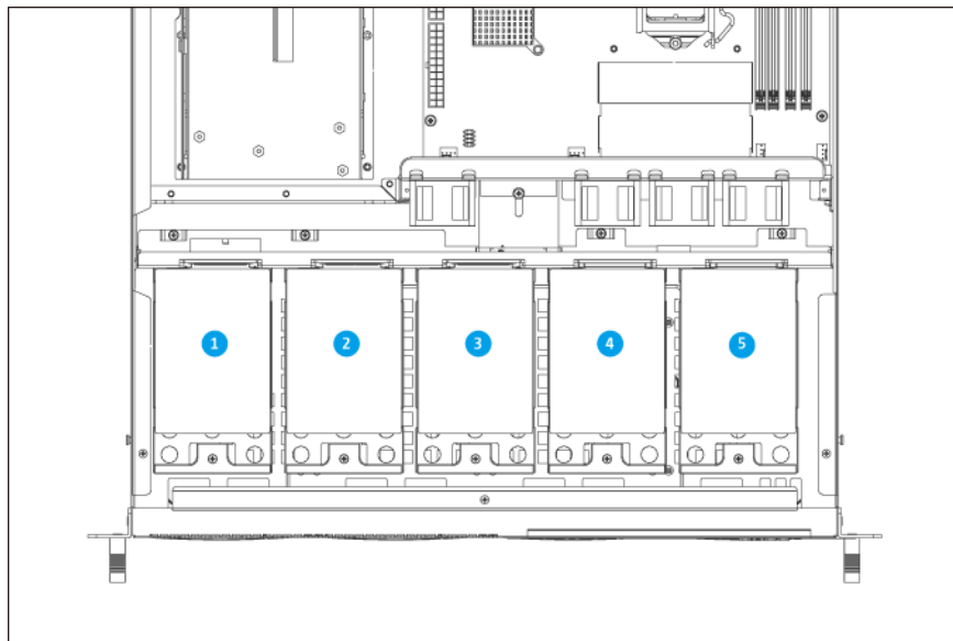
2.5 吋硬碟插槽
